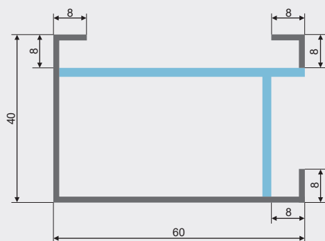
Spessore parete 2 mm Spessore parete 3 mm
