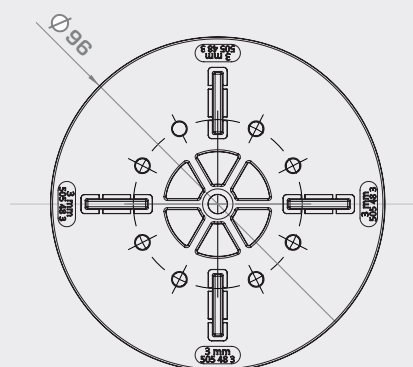
TERRASYS supporto a scorrimento per binario
